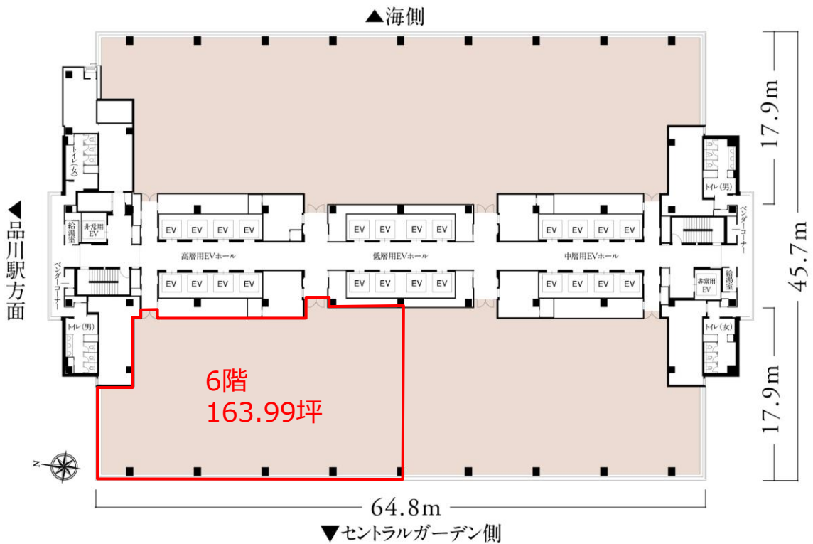
基準階平面図
