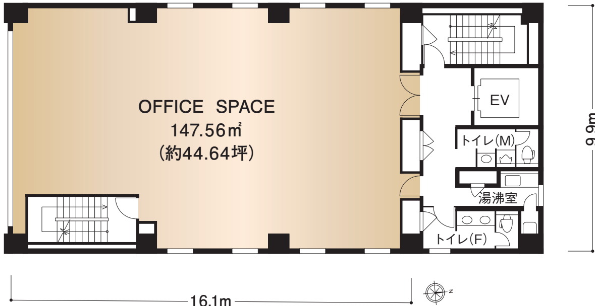
6階平面図
