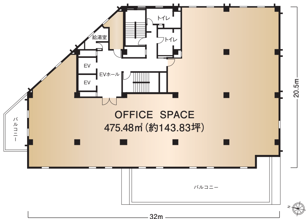
7 階平面図
