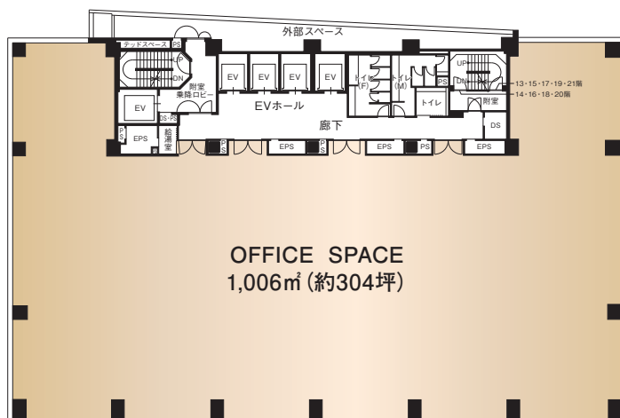
15階平面図
