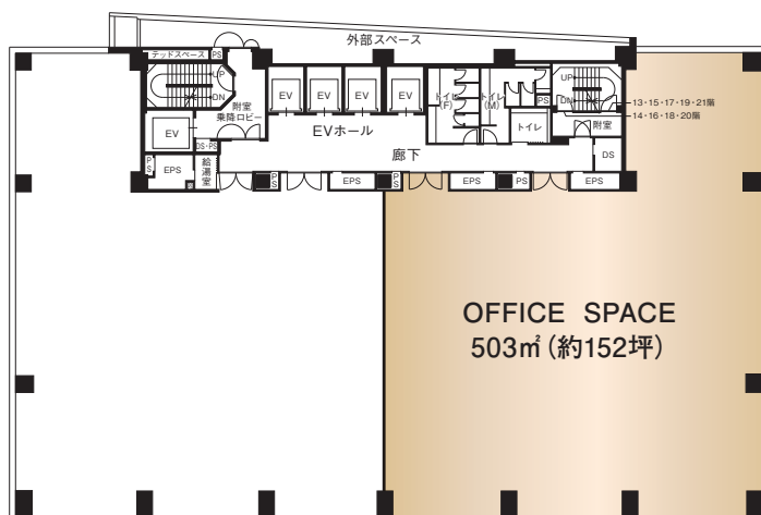
13階平面図
